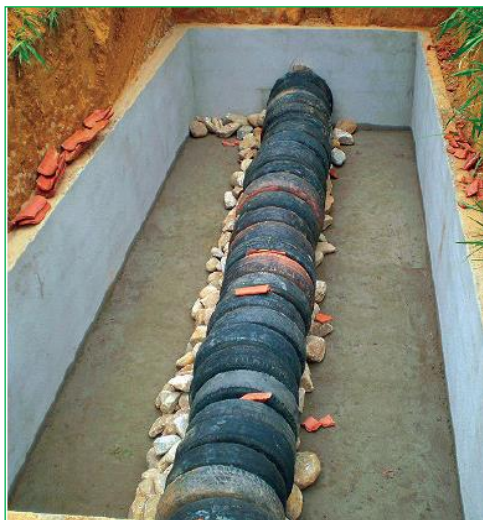
Figura 4.2 – TEvap – Trincheira impermeabilizada e câmara de digestão montada. Fonte: Leal, 2014.
