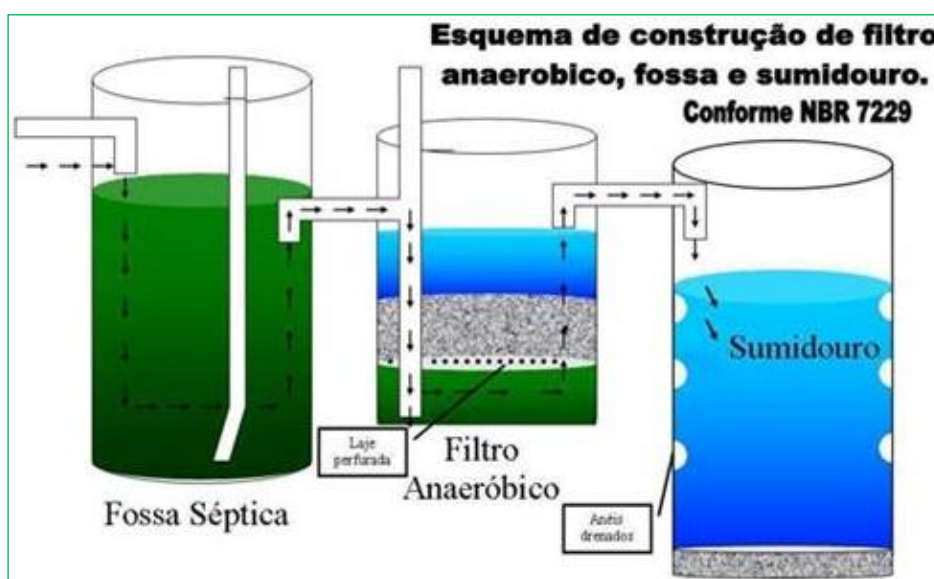
Figura 4.1 – Esquema do conjunto Fossa-filtro-sumidouro.
