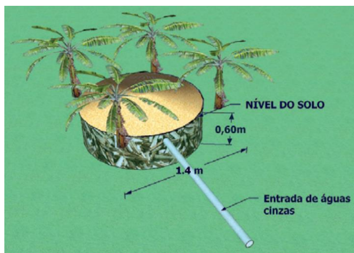
Figura 4.13 – Desenho esquemático do círculo de bananeiras.
