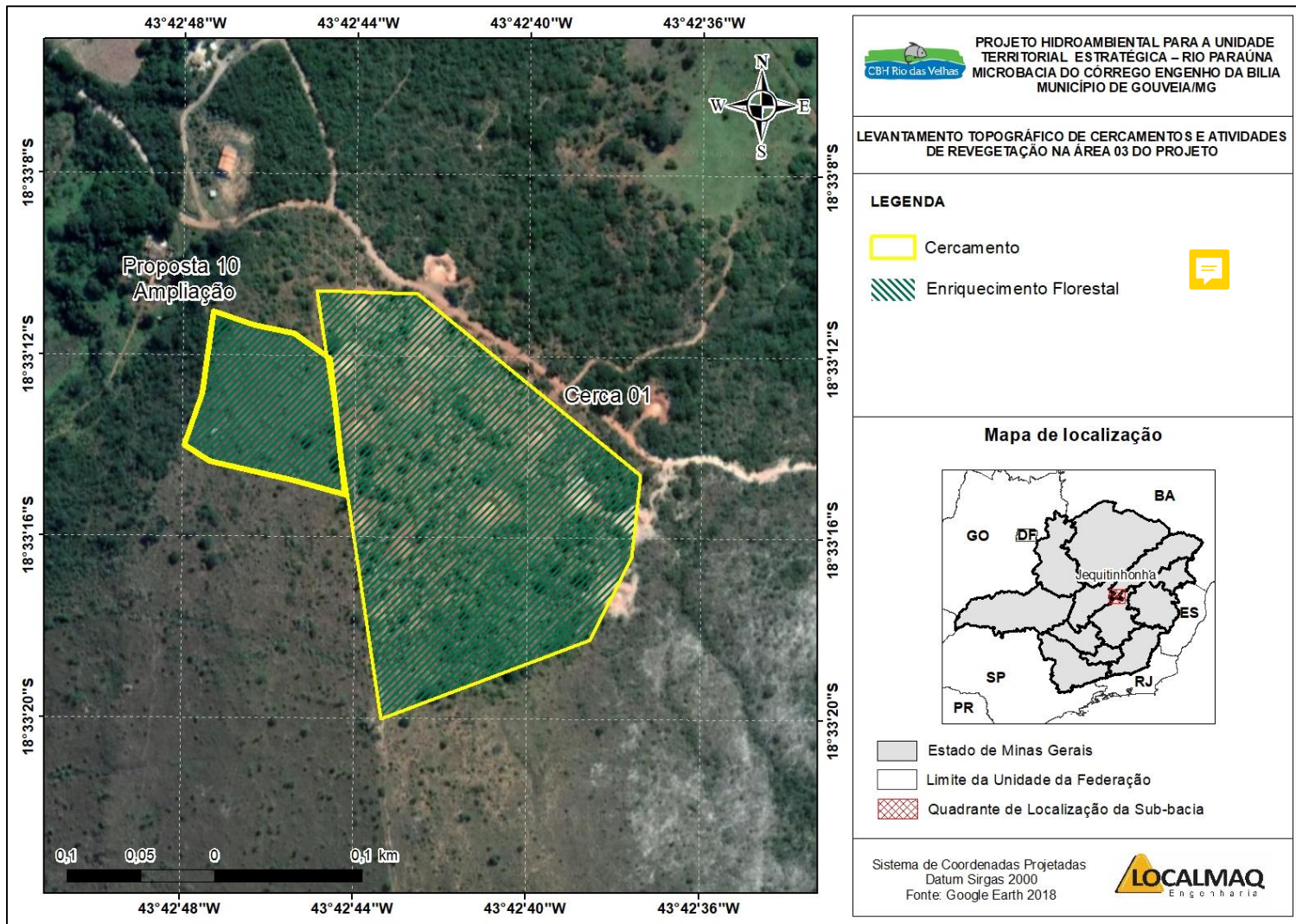
Figura 5 – Levantamento topográfico do cercamento e atividades de revegetação realizado na segunda etapa de Topografia, na área 3 do projeto Fonte: LOCALMAQ, 2018
