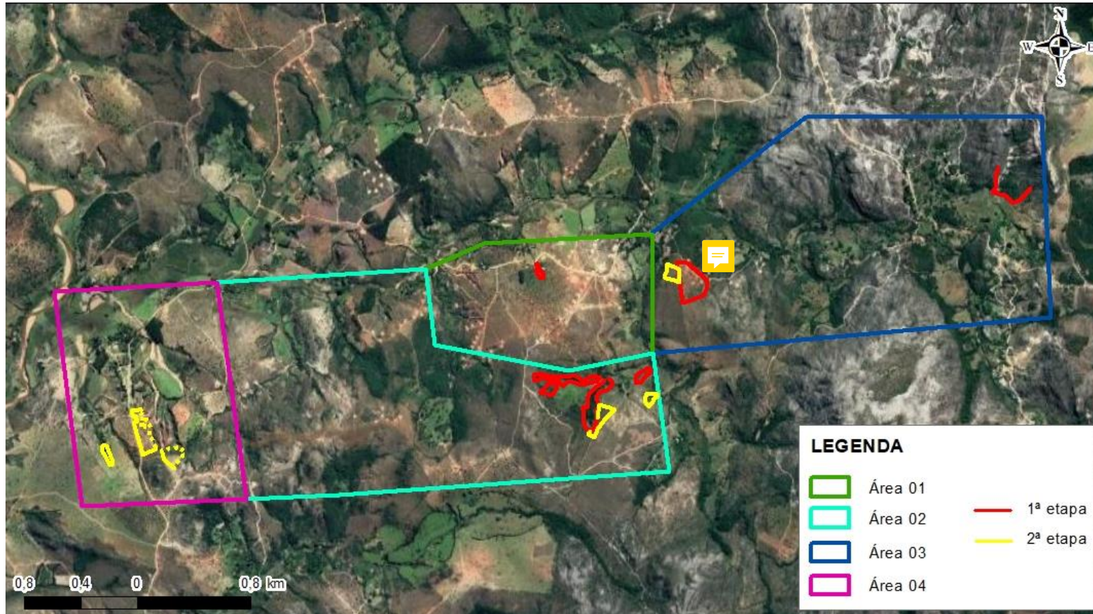
Figura 9. Levantamento Topográfico geral de cercamentos e atividades de revegetação ao longo da área de atuação do projeto
