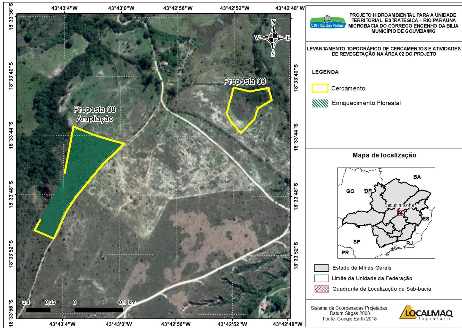
Figura 4 – Levantamento topográfico do cercamento e atividades de revegetação realizado na segunda etapa de Topografia, na área 2 do projeto Fonte: LOCALMAQ, 2018
