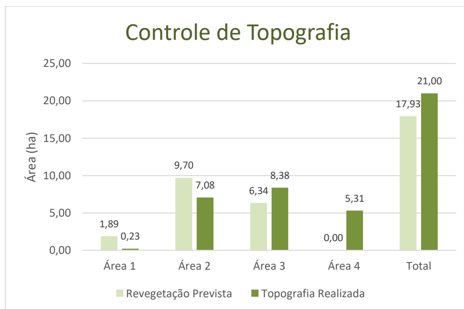
Figura 8 - Locação topográfica de revegetação prevista e realizada nas áreas de atuação do projeto Fonte: LOCALMAQ, 2018
