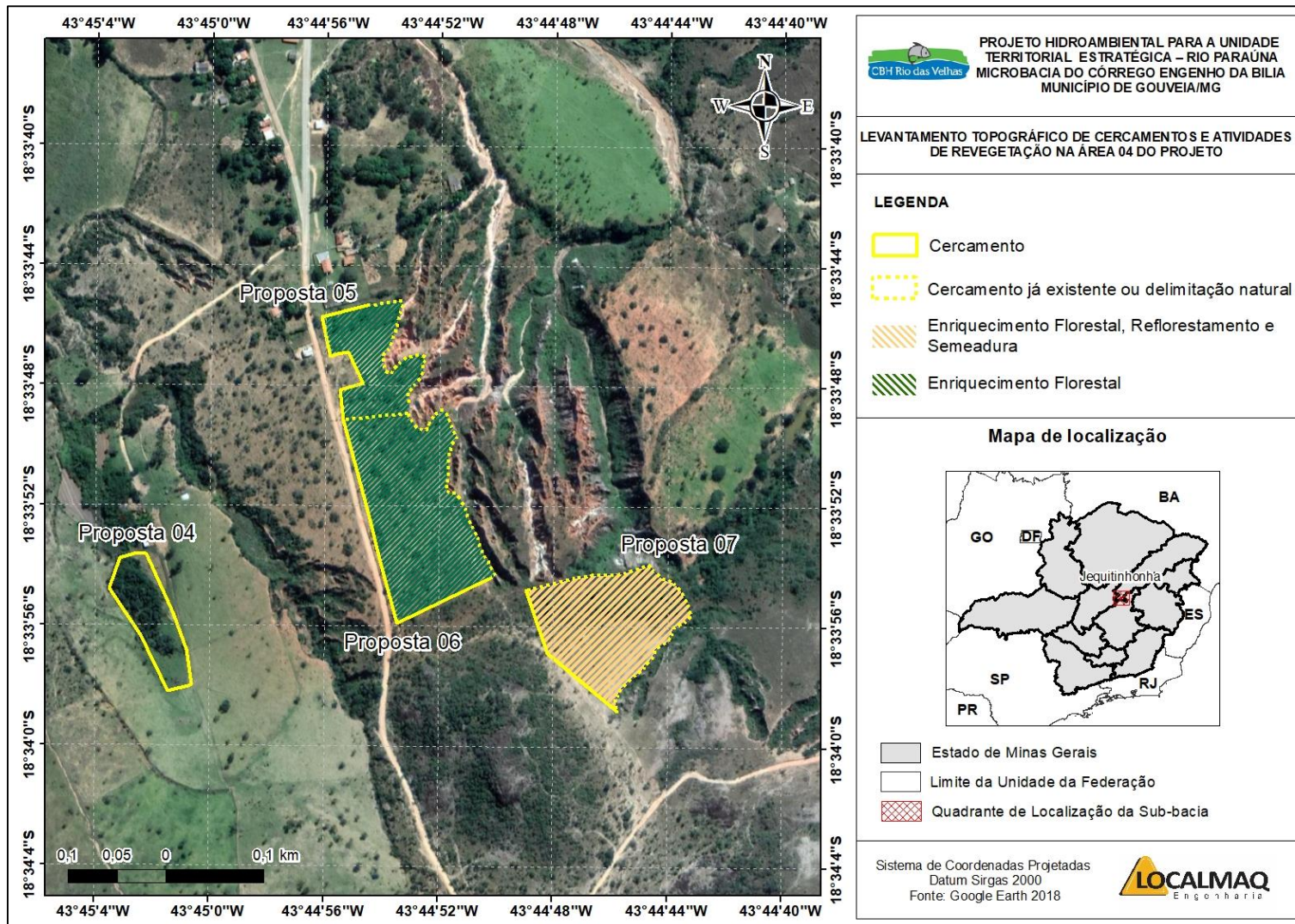
Figura 6 – Levantamento topográfico do cercamento e atividades de revegetação realizado na segunda etapa de Topografia, na área 4 do projeto Fonte: LOCALMAQ, 2018
