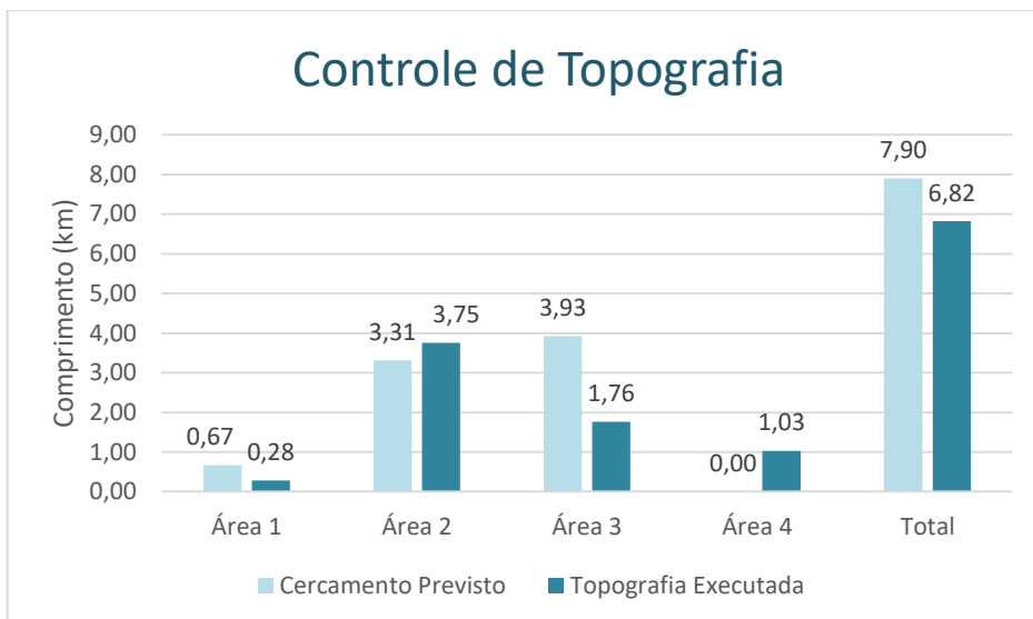
Figura 7 - Locação topográfica de cercamento previsto e realizado nas áreas de atuação do projeto Fonte: LOCALMAQ, 2018
